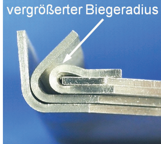
Bild 1: Hohlfalz (Prozessfolge - Abkanten, Vor- und Fertigfalzen)
