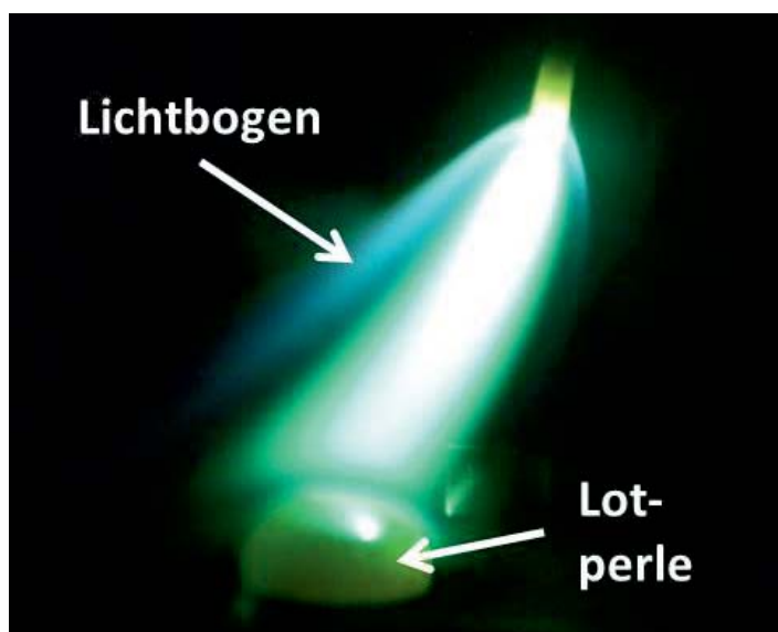
Erschmelzen einer Lotlegierungsperte im Lichtbogenofen
